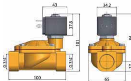
Massbild 046
