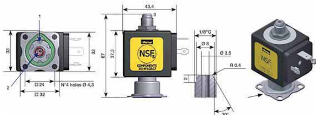
Massbild 072
