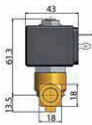
Massbild 008
