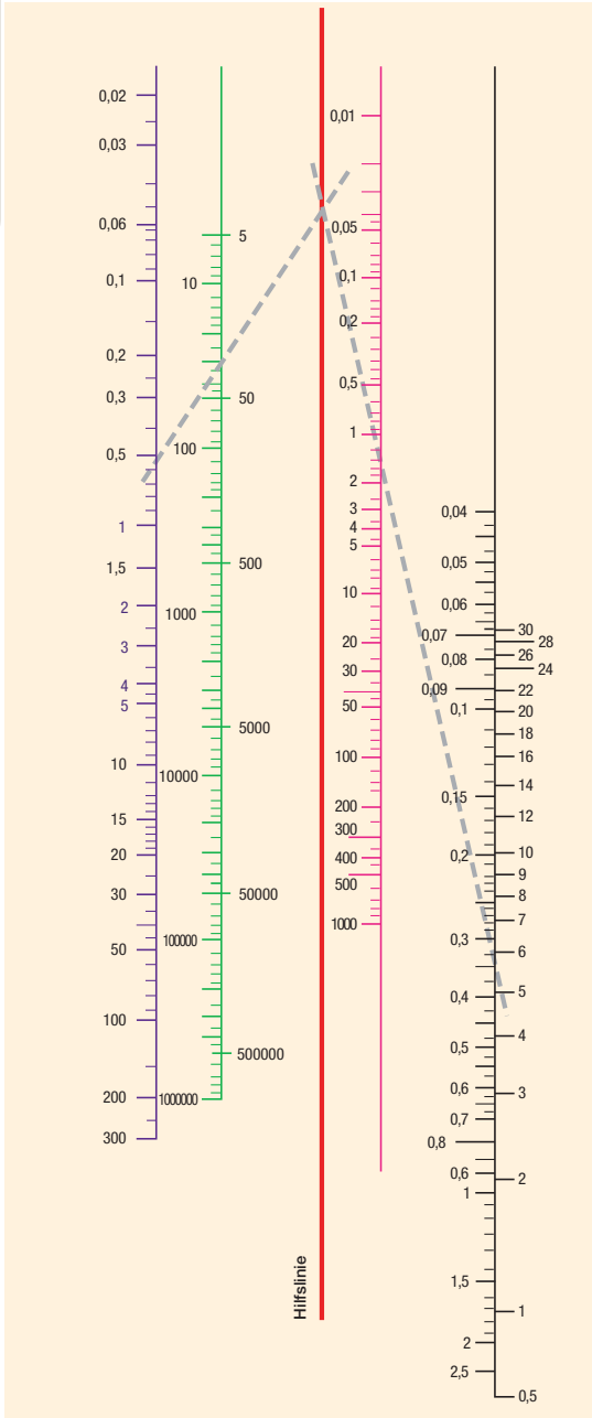
Diagramm 3 für trockengesättigten Dampf Dampfdaten (trockengesättigt)
