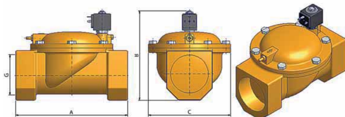
Massbild 063
