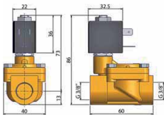
Massbild 054
