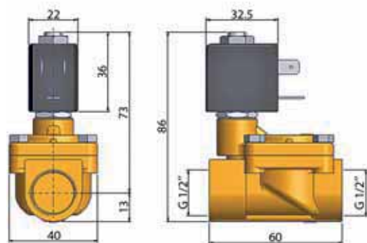
Massbild 053
