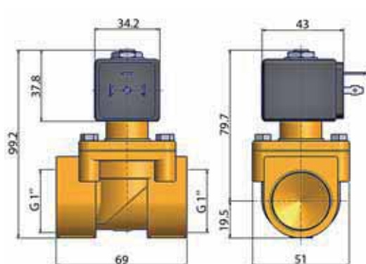
Massbild 040
