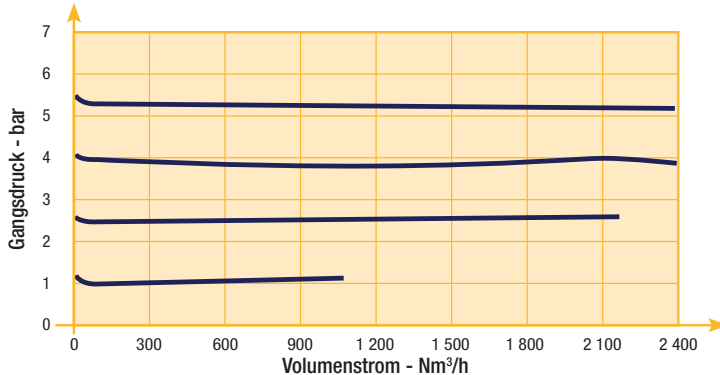
Fließkurve 2"
