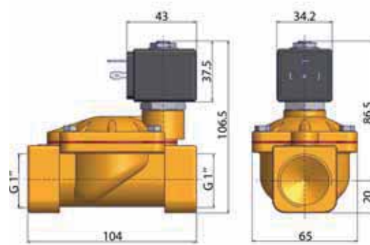
Massbild 047
