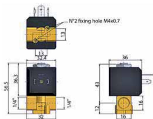
Massbild 014
