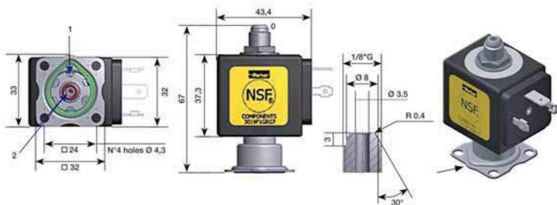
Massbild 072
